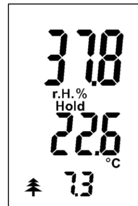
Abbildung 5-15: Messmenü «Holzfeuchtegleichgewicht, UGL»
