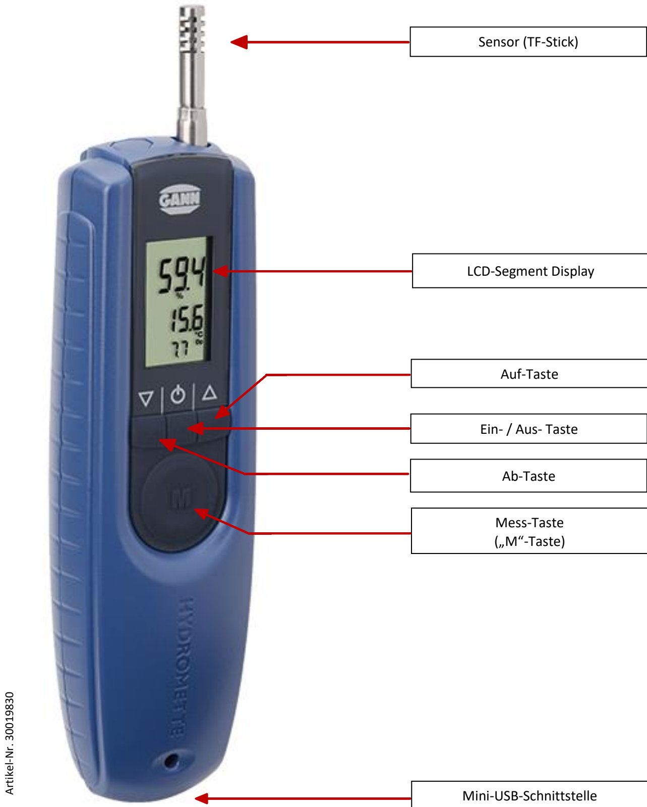
Abbildung 5-1: Ansicht der Hydromette BL Compact TF 3
