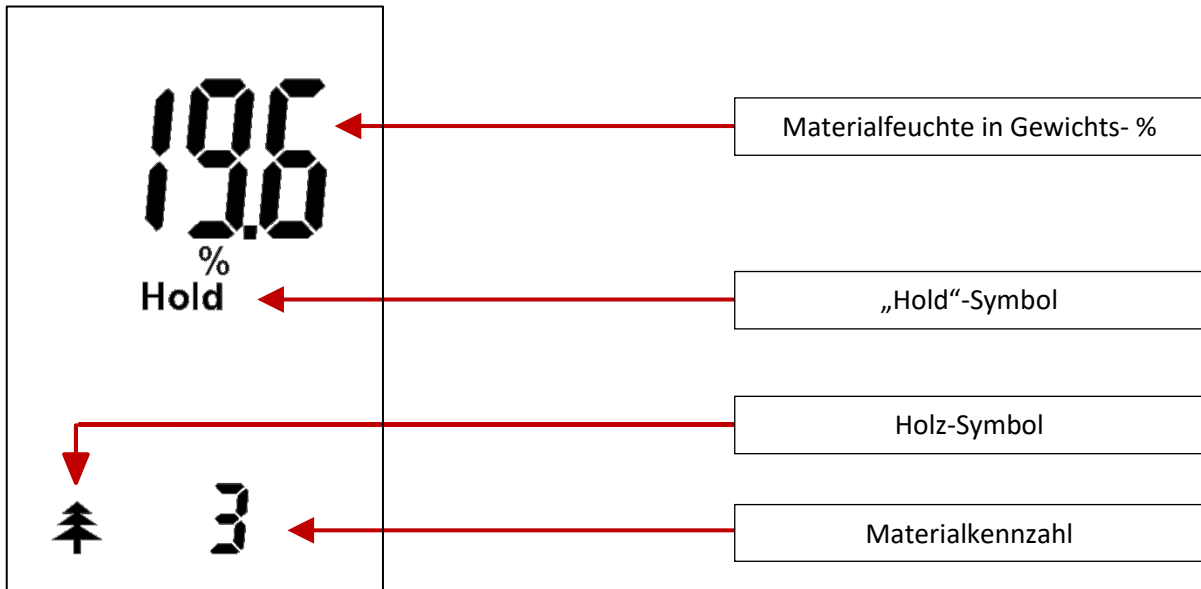
Abbildung 5-2: Symbole Hauptmenü
